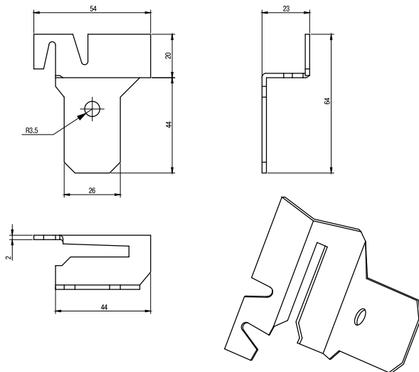
Рисунок 1 – Габаритные размеры
